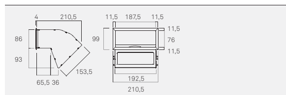
D1005 Difusor de salida de aire doble
