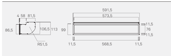
D0015 Difusor de entrada de aire cuádruple
