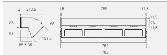
D1015 Difusor de salida de aire cuádruple
