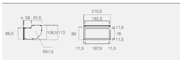
D0005 Difusor de entrada de aire doble
