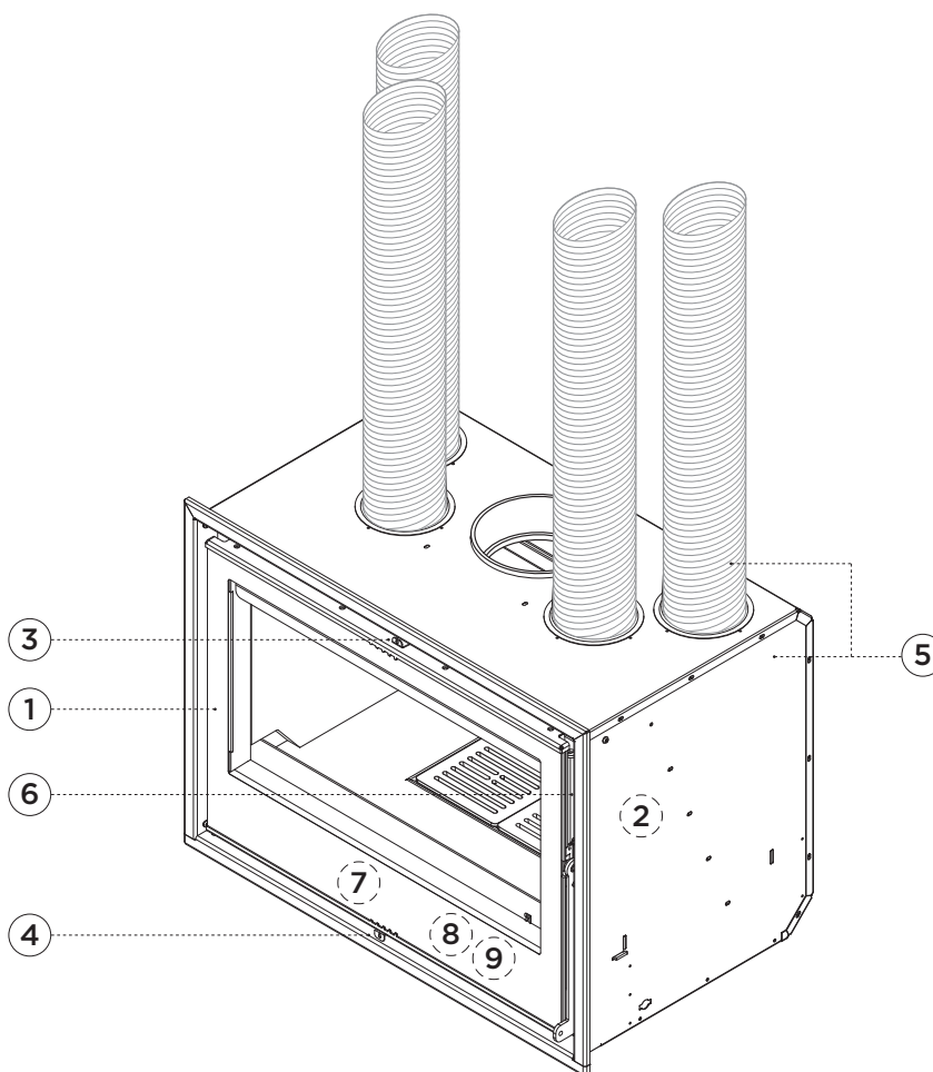
* Croquis explicativo Modelo RCr80 graffiti
