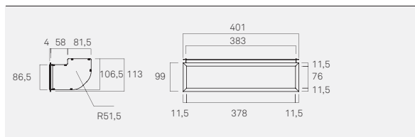
D0010 Difusor de entrada de aire triple
