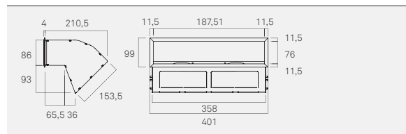
D1010 Difusor de salida de aire triple
