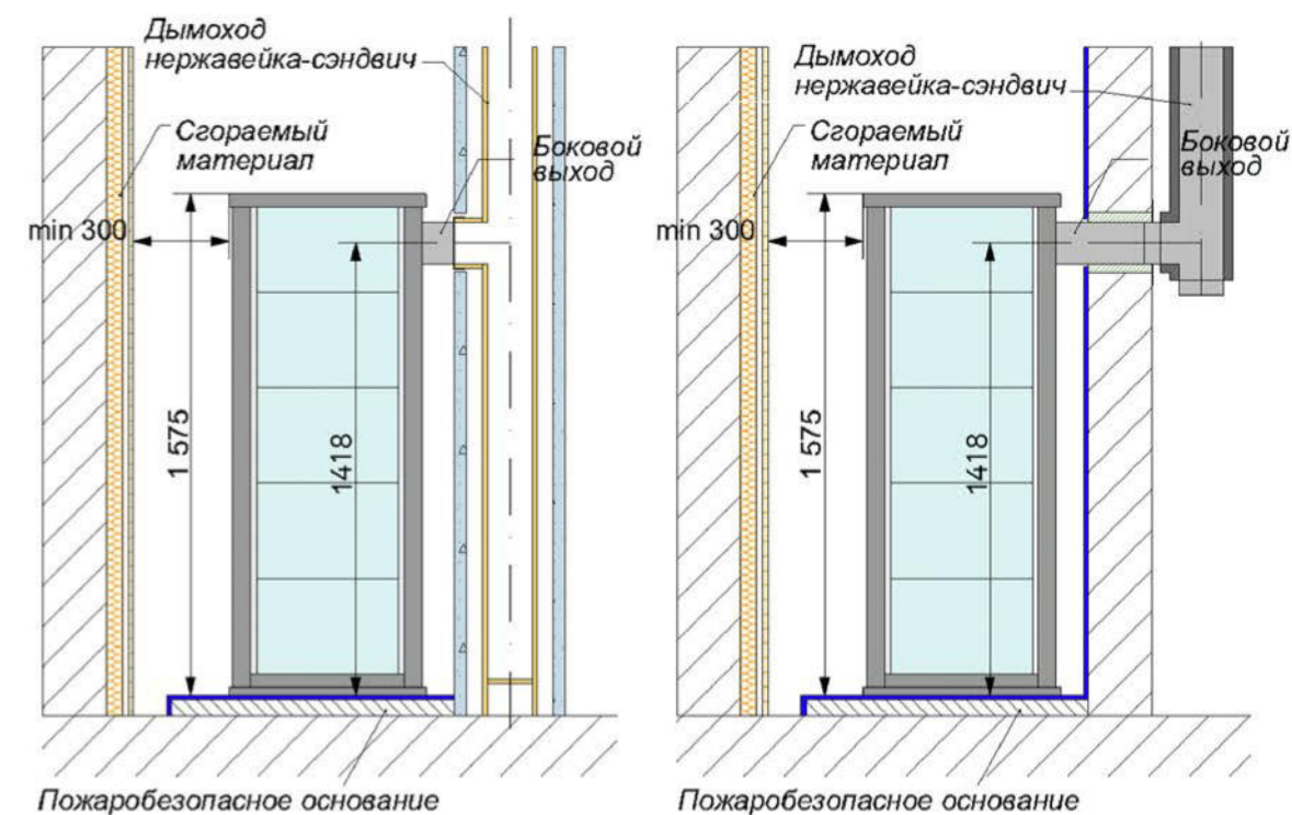
Схематичный чертеж подключения KLV-RT-35RV 310s к дымоходу
