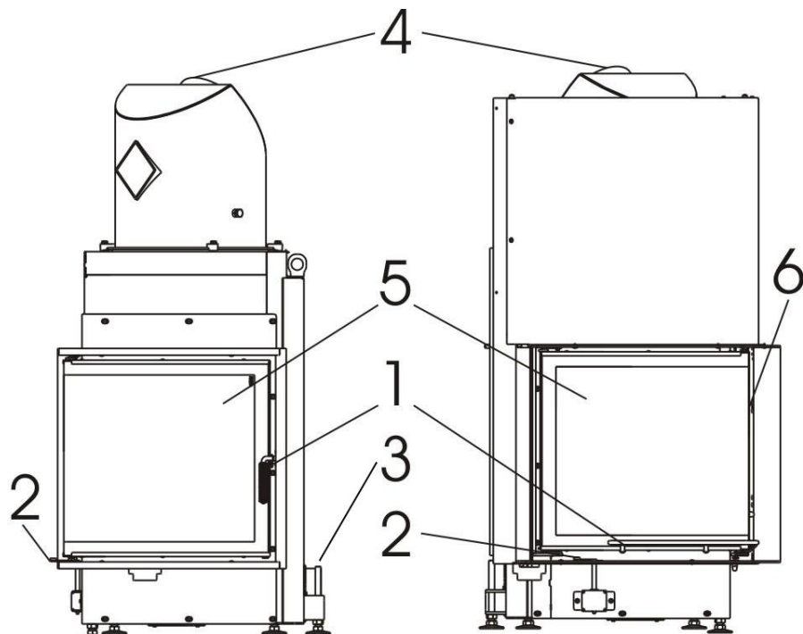
Иллюстрация 2: Компоненты каминных топок "Eck" (схематическое изображение)
