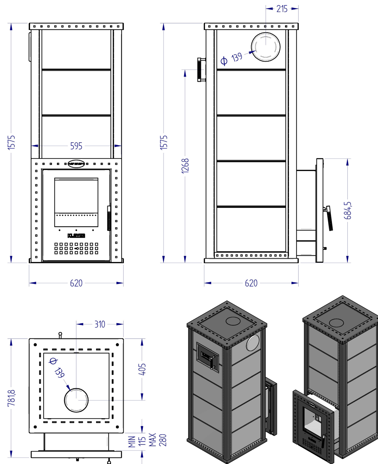
Габаритные размеры – Печь KLV-RT-35RV
