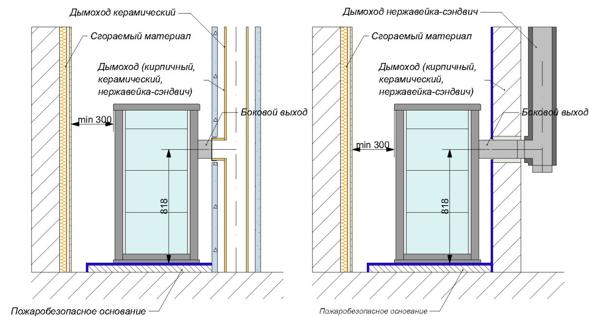
Схематичный чертеж подключения KLV-RT-35P к дымоходу
