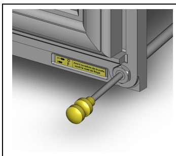
Механизм регулировки тяговой заслонки: открытое положение
