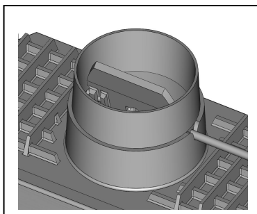
Механизм регулировки тяговой заслонки: открытое положение
